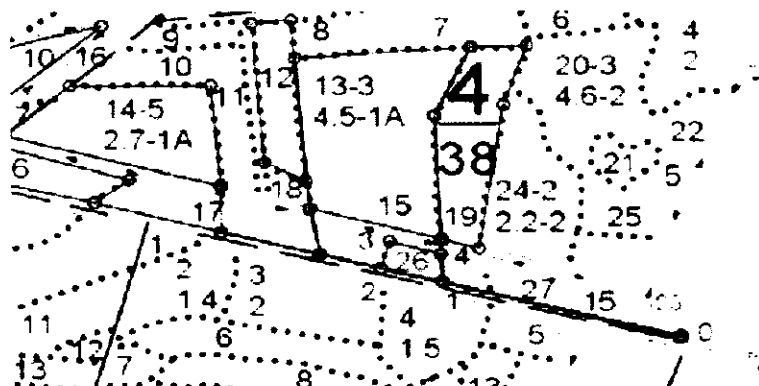
Абрис участка М 1:10000
