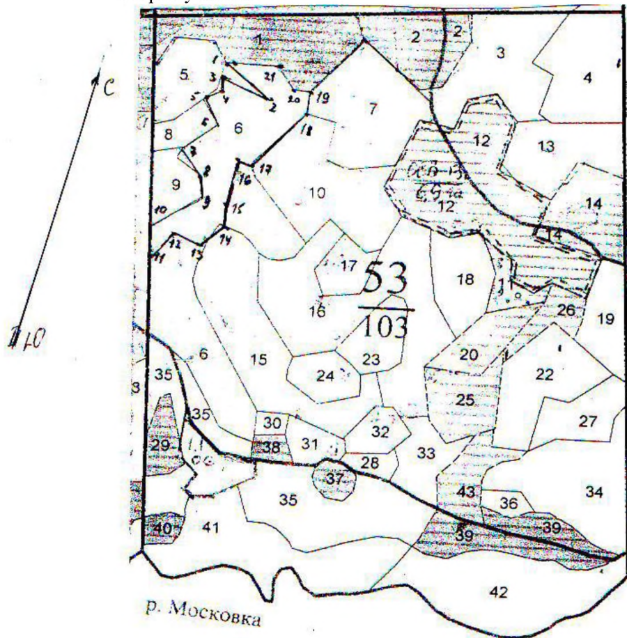
Абрис участка
