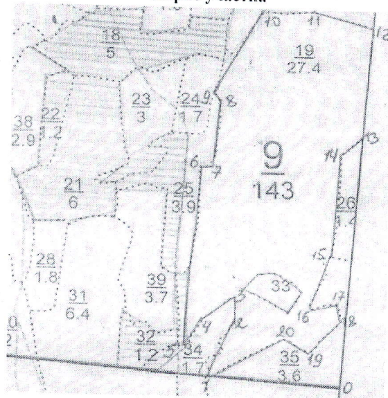
Абрис участка
