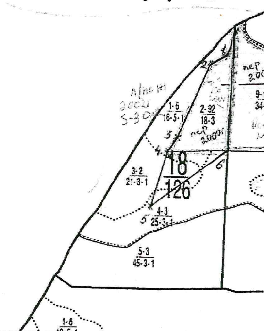
Абрис участка
